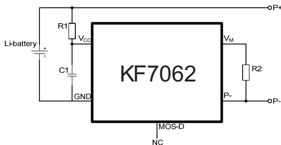
图-1 KF7062 典型应用电路图
